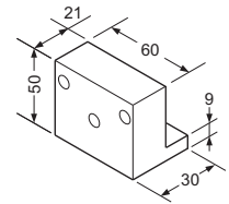
Anschlagplatte Artikel-Nr.: 100.004
